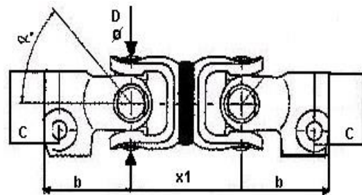
JUNTA DOBLE CON ACOPLAMIENTO ABIERTO
