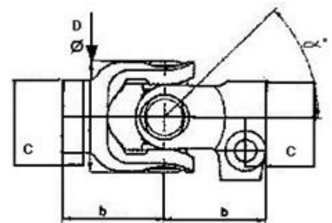
JUNTA SIMPLE CON ACOPLAMIENTO ABIERTO
