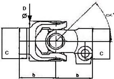
JUNTA SIMPLE CON ACOPLAMIENTO ABIERTO
