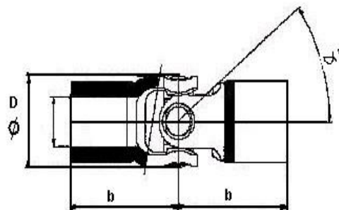
JUNTA SIMPLE A CRUCETA
