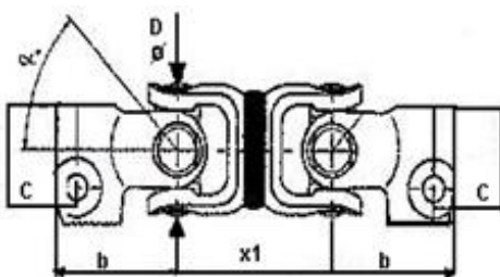
JUNTA DOBLE CON ACOPLAMIENTO ABIERTO
