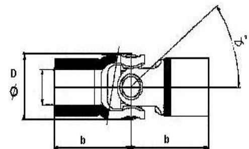
JUNTA SIMPLE A CRUZETA
